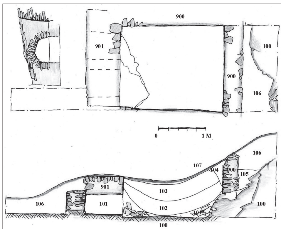
Obr. 1: Holštejn, půdorys a řez vápenickou pecí. 900 obvodové kamenné zdivo pece, 901 zdivo s dvojicí tahových kanálů, 100 skalní podloží, 101 destrukce tělesa pece po jejím zániku, 102, 103 a 106 postupně vznikající zásyp terénní deprese v místě pece, 104 recentní výkop zřejmě staršího „výzkumu“, 105 dorovnávká mezi vyzdívkou pece a skalním podložím, 107 lesní humus
