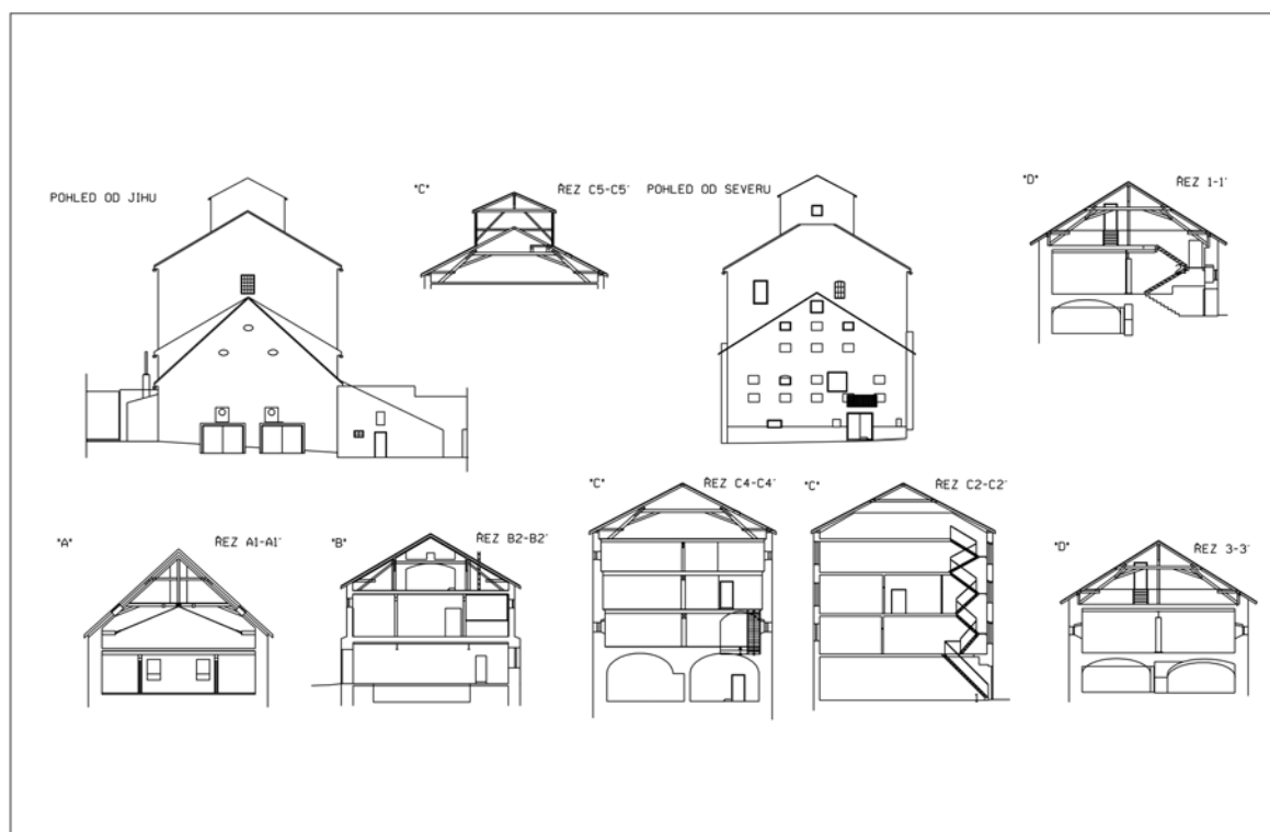
Obr. 11 Nárys severního a jižního průčelí traktu bývalého pivovaru. Řezy jednotlivými objekty
